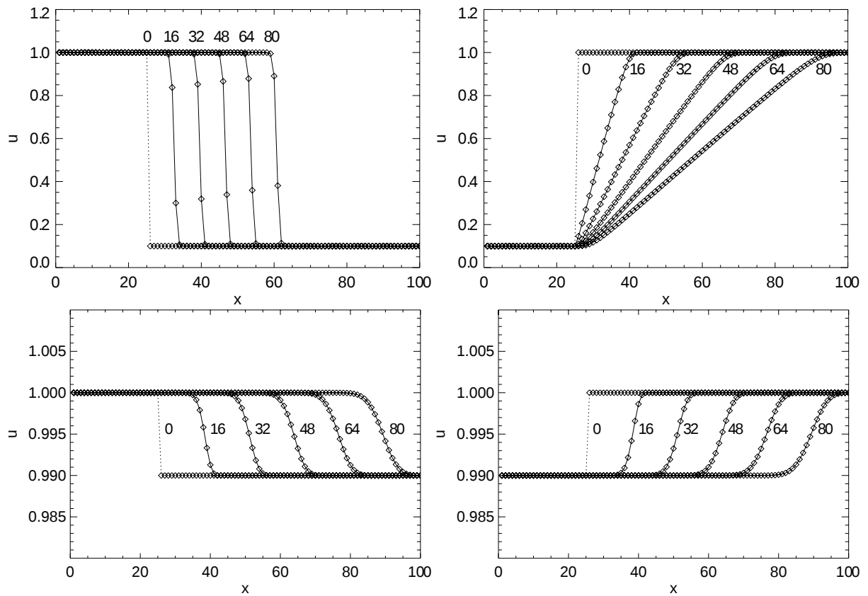
図 2.4: 非粘性バーガース方程式のリーマン問題。(左) u_L = 1, u_R = 0.1 の場合、衝撃波型 ( t = 0.8 \times [0, 16, 32, 48, 64, 80] )。 (右) u_L = 0.1, u_R = 1 の場合、希薄波型 ( t = 0.8 \times [0, 16, 32, 48, 64, 80] )。下はそれぞれ、振幅が微小で線形な系としてふるまう場合で、(左) u_L = 1, u_R = 0.99 の場合と (右) u_L = 0.99, u_R = 1 の場合。
