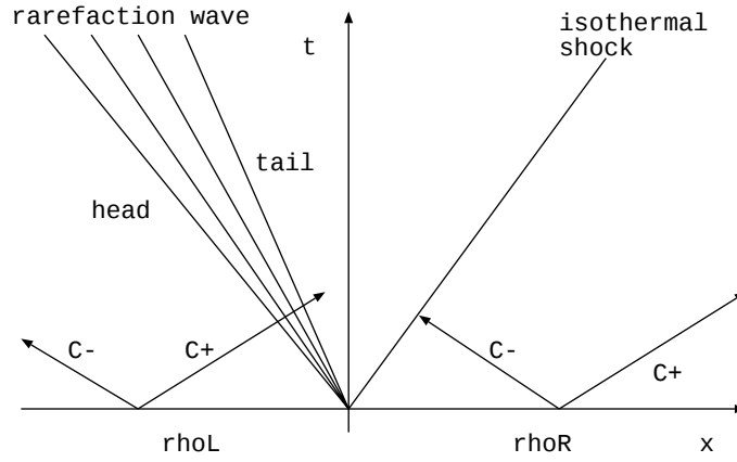
図 2.6: 等温の衝撃波管問題。
