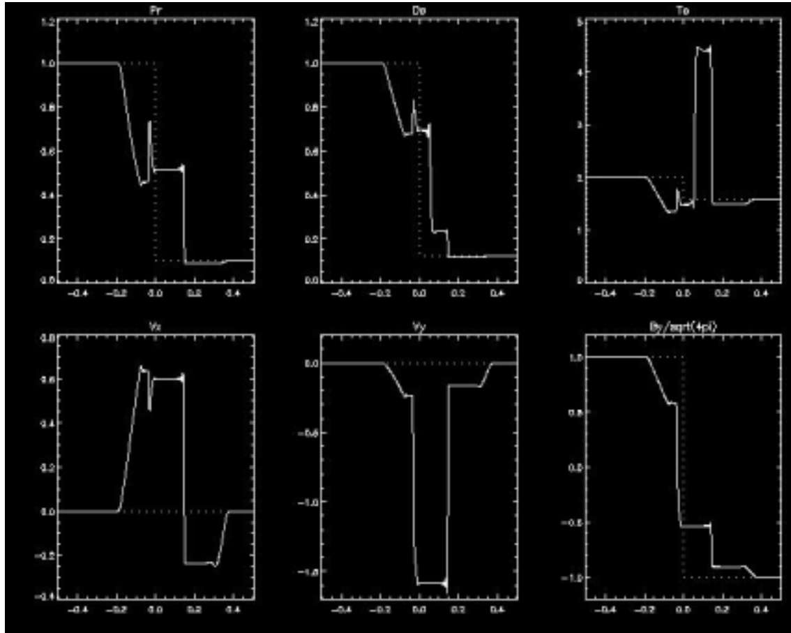
図 4: md_mhdshktb の結果
